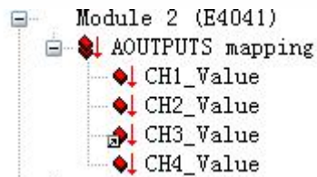
图 13 模块 (E4041) 地址映射 (模块位置不同 SDO 参数号也不一样从 8010 开始)
