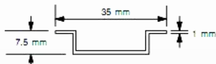
图 2 DIN 导轨
